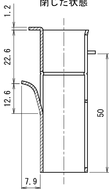
A-A断面図
