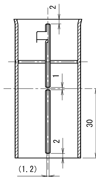
B-B断面図
